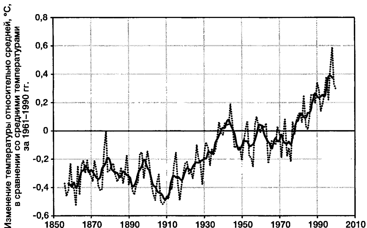
Рис. 3.27. Рост мировой температуры
