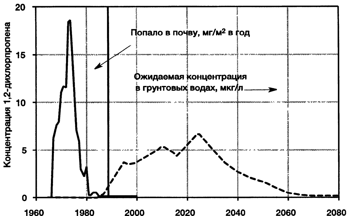
Рис. 4.10. Медленное проникновение 1,2-дихлорпропена в грунтовые воды. Дезинфицирующий химикат для обработки почв дихлорпропеном широко применялся в Нидерландах в семидесятые годы, пока его использование не было ограничено, а затем окончательно запрещено в 1990 г. В результате концентрация дихлорпропена в верхних слоях почвы сельскохозяйственных угодий резко уменьшилась. Расчеты, проведенные в 1991 г., показывают, что концентрация этого соединения в грунтовых водах достигнет максимума не раньше 2020 г. и что в воде даже во второй половине XXI в. будут присутствовать существенные количества этого химиката. (Источник: N.L. van der Noot.)
