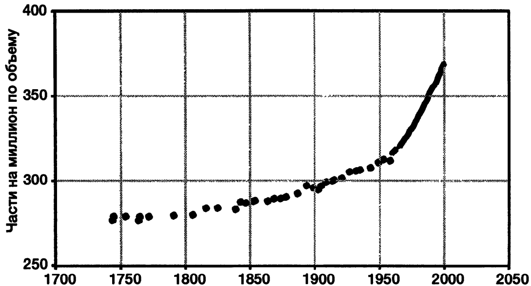
Рис. 1.3. Концентрация в атмосфере диоксида углерода
