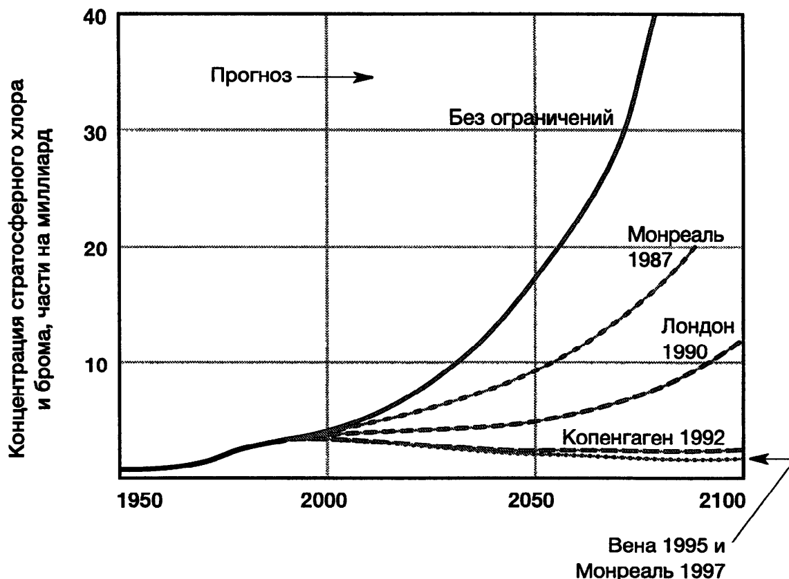
Рис. 5.6. Предполагаемое увеличение концентраций стратосферного неорганического хлора и брома в результате выбросов ХФУ
