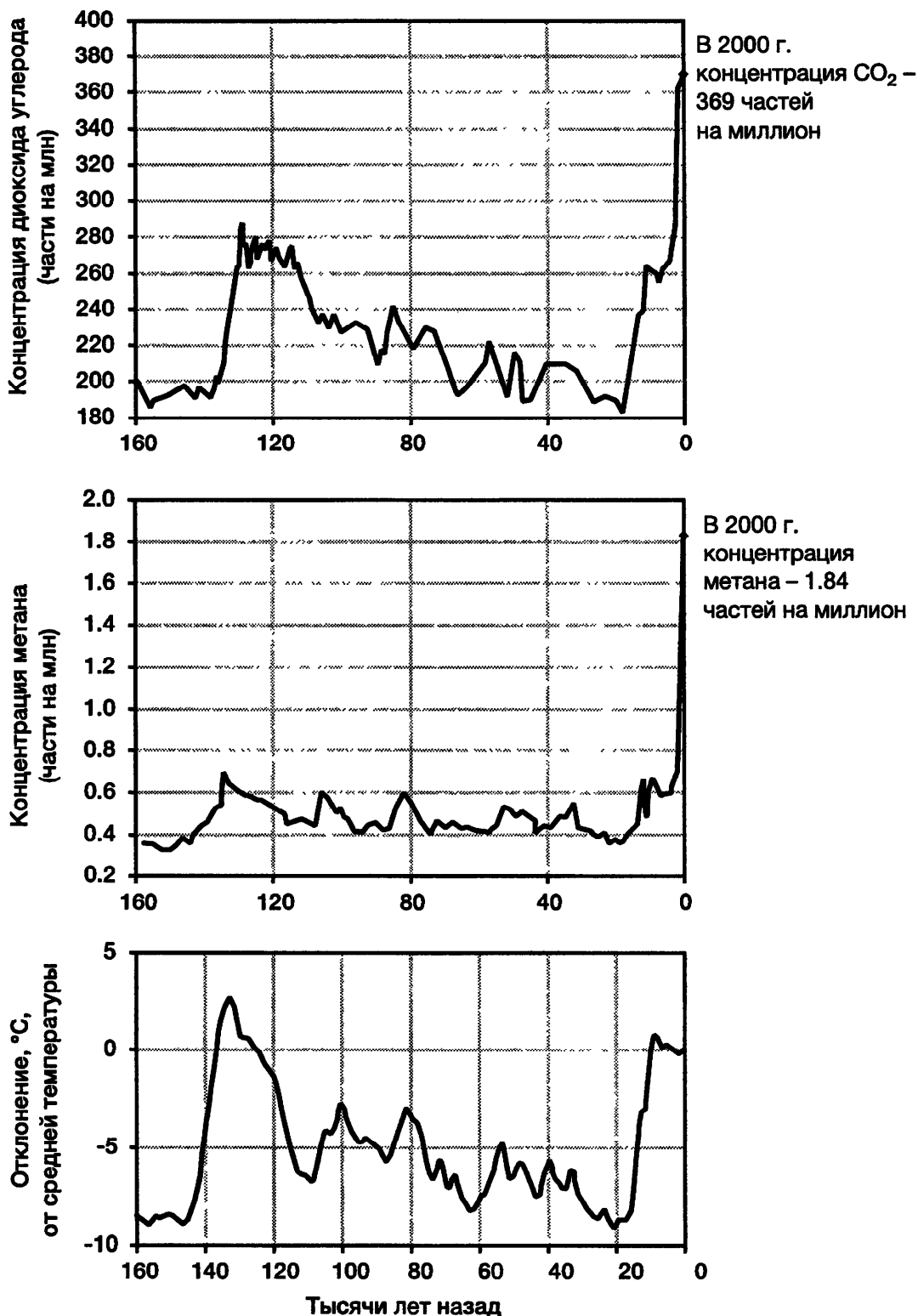
Рис. 3.29. Парниковые газы и средняя глобальная температура за прошедшие 160 тыс. лет
