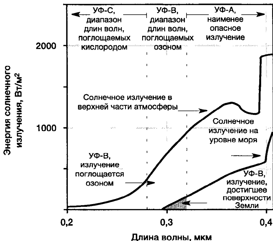
Рис. 5.2. Поглощение излучения в атмосфере
