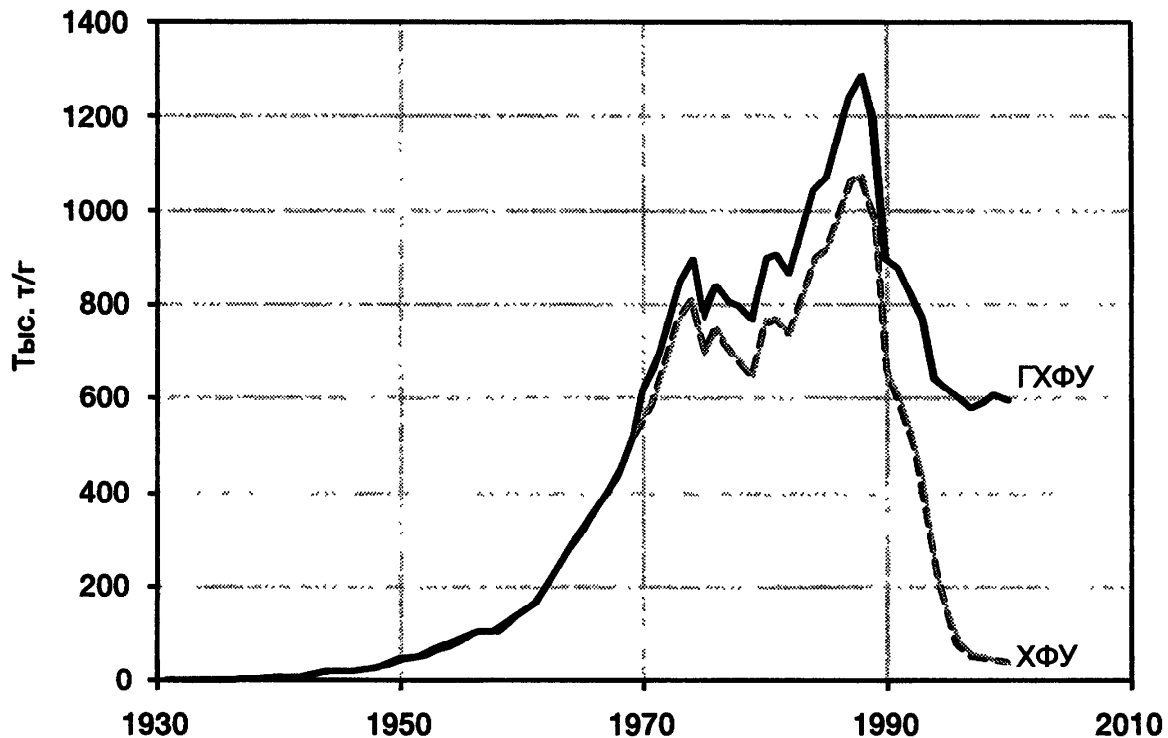
Рис. 5.1. Мировое производство хлорфторуглеродов
