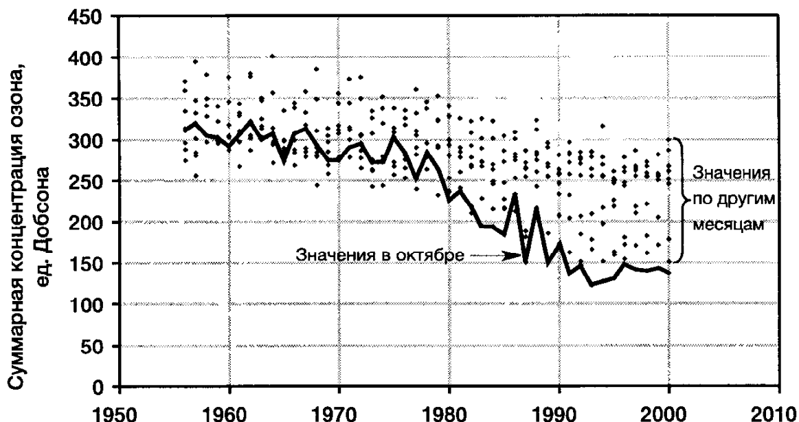
Рис. 5.4. Измерение концентрации озона, станция Халли, Антарктида
