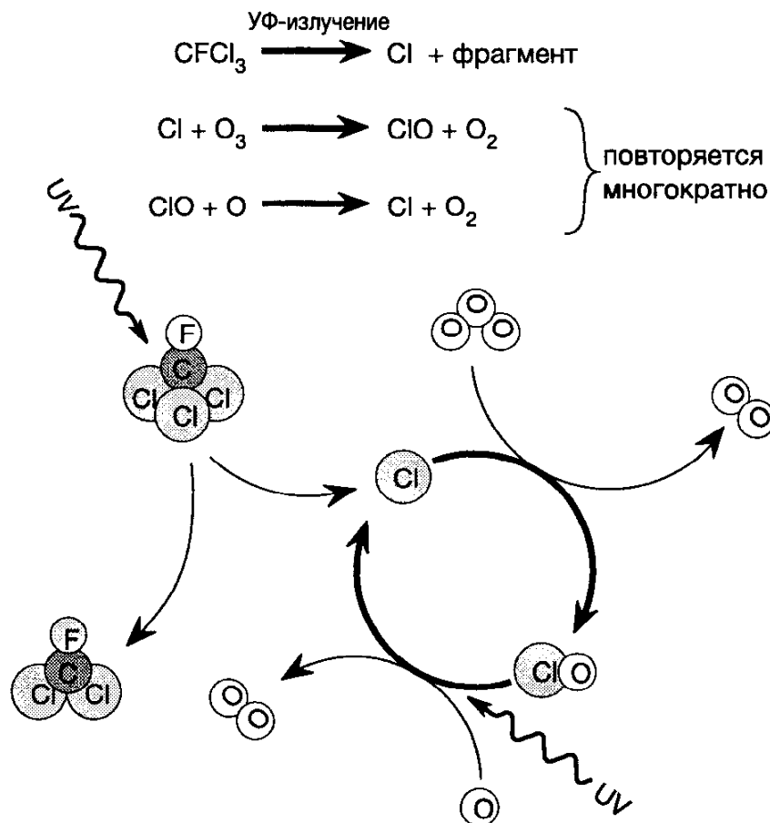
Рис. 5.3. Как ХФУ разрушают стратосферный озон
