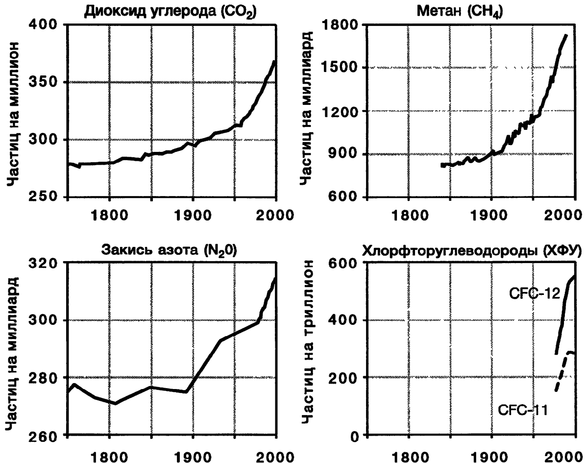
Рис. 3.26. Концентрации глобальных парниковых газов
